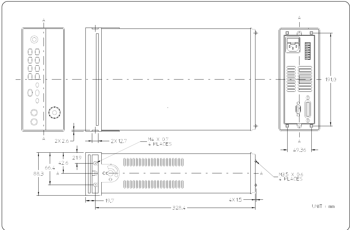
Figura 8-2. Dimensiones para el montaje en bastidor
